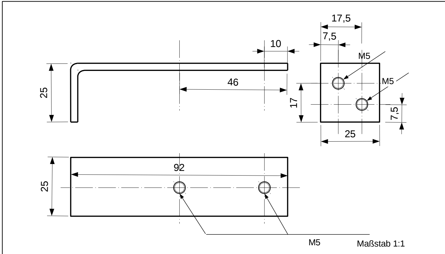
Bild 1: Halter
